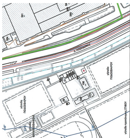
ΠΕΡΙΟΧΗ Δ_ΚΛΙΜΑΚΑ 1:200
